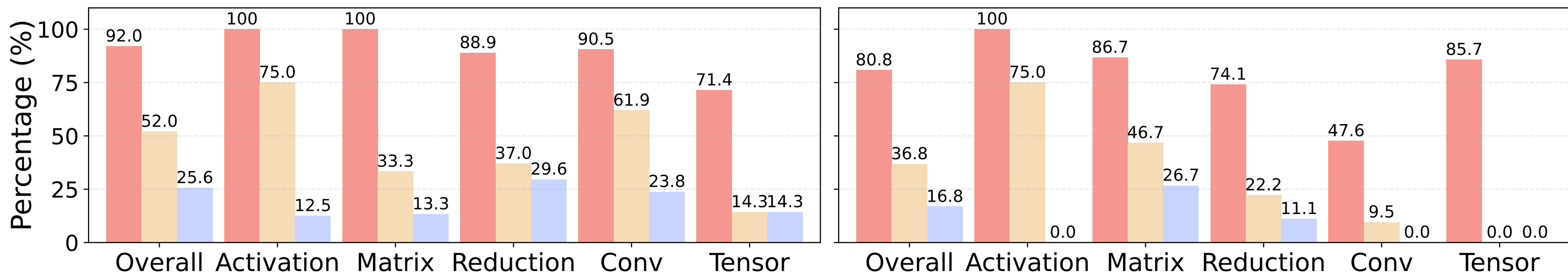
(b) NCNN
